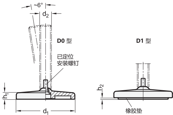
螺杆的款式
