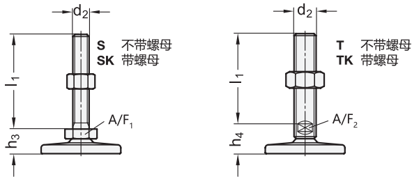
螺杆的款式
